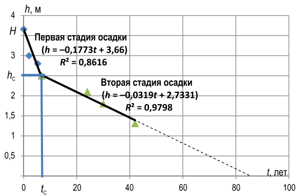
Рис. 1. Осадку осушенной торфяно-болотной почвы Флориды (США), по данным Р. Эллисон [2] (штрихами показана прогнозируемая экстраполяция линейной зависимости, проведенной по четырем опытным точкам)
