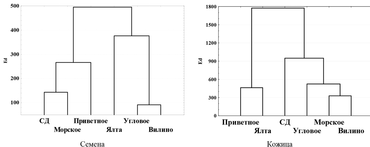
Рис. 3. Результаты кластерного анализа винограда из различных географических объектов по комплексу фенольных антиоксидантов в структурных частях ягод (СД – с. Солнечная Долина)
