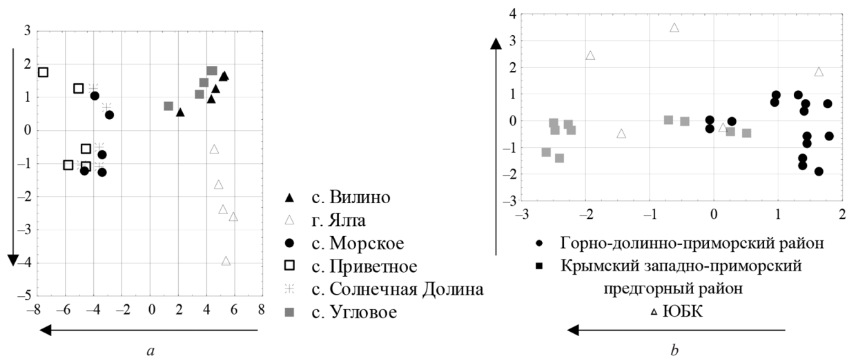
Рис. 2. Результаты дискриминантного анализа территорий произрастания винограда по теплоресурсам: a – по географическим объектам и влагообеспеченности; b – по виноградарским районам
