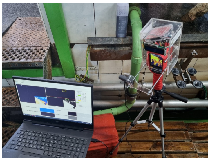
Рис. 1. Макетный образец устройства биометрической идентификации предмаститного состояния вымени коров дойного стада
