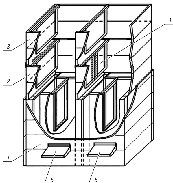
Рис. 1. Схема двухблочного пчелиного улья с комбинированной технологической перегородкой
