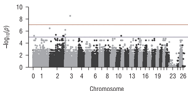
Рис. 1. Манхэттенский график результатов GWAS с набором значений -\log_{10}(p) для исследуемых SNP. Синей линией обозначен порог различий с ожидаемой достоверностью различий при значении -\log_{10}(p) = 5 , красной линией – порог достоверности различий при значении -\log_{10}(p) = 7
